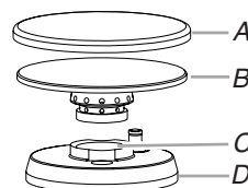
A. Chapeau de brûleur B. Tête de brûleur C. Ouverture de gaz D. Base du brûleur
